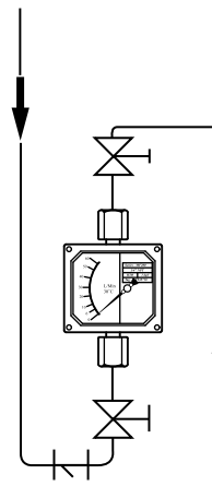
Установка в вертикальную линию, поток сверху вниз
