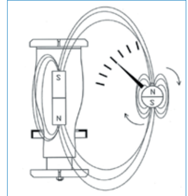
Принципиальная схема
